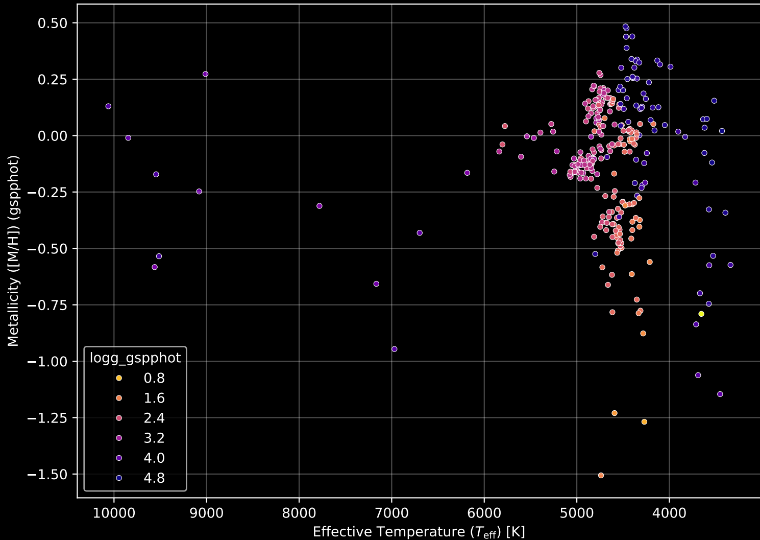
APOGEE DR17 Field: [169+18_btx] Stellar Population Parameters (n= 303)
